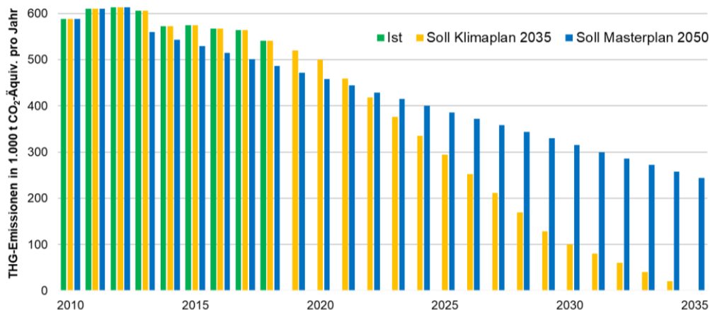
Abb. 3: Notwendiger CO 2 -Minderungspfad der Stadt Kempten, um Treibhausgas-Neutralität bis 2035 in Anlehnung an den 1,5 °C-Klimaplan von GermanZero [4] zu erreichen, sowie der ursprüngliche Minderungspfad bis 2050 aus dem Masterplan „100 % Klimaschutz“ und die aktuelle Entwicklung der Treibhausgas-Emissionen der Stadt Kempten.
