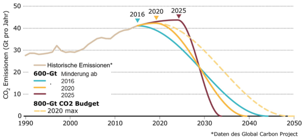
Abb. 1: Notwendige Entwicklungspfade der weltweiten THG-Emissionen zur Einhaltung des 600-Gt-Budgets in Abhängigkeit des Beginns signifikanter Minderungen [11] .
