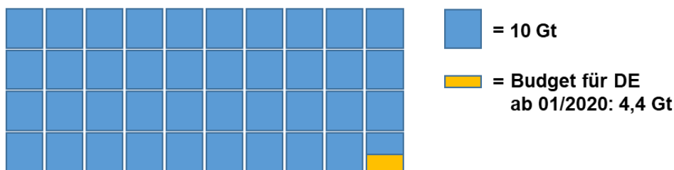
Abb. 2: Global und für Deutschland noch verfügbares Emissionsbudget ab 2020, um die globale Erwärmung mit einer 2/3 Wahrscheinlichkeit auf 1,5 °C zu begrenzen (Daten: IPCC [9] ).
